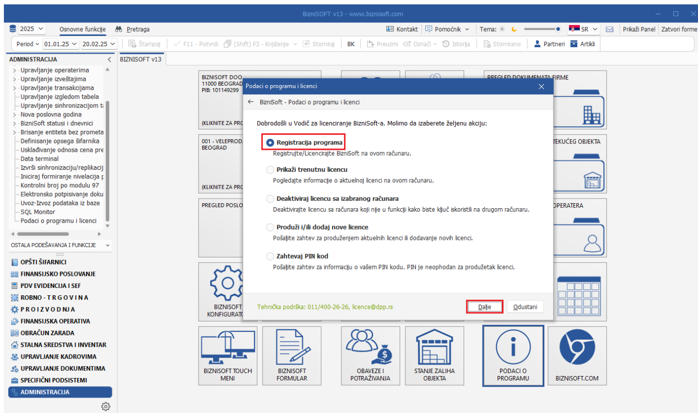
Slika 3 – Registracija programa
